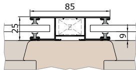
Sloupek s vodicí lištou K85V
