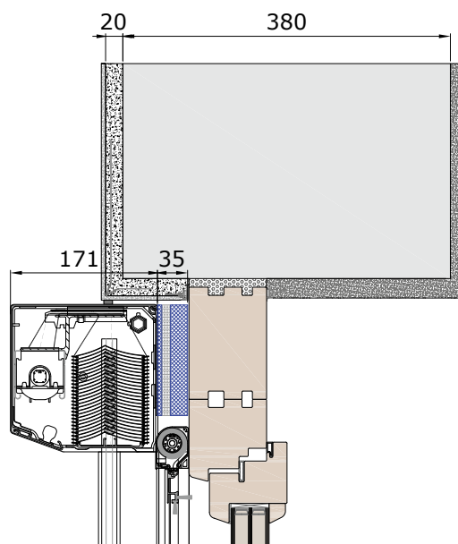
S rámovým zdvojením a zateplením překlady. VORO RAFF (80D) RetroLux s kombinovanou rolo sítí.
