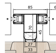
Sloupek s ED85V
